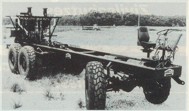
Stabile Titan-Fahrzeugrahmen für Feuerwehrfahrzeuge.
