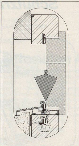
Schwellenschiene Hebgo Nr. 163 EP-Gummidichtung Hebgo Nr. 633
