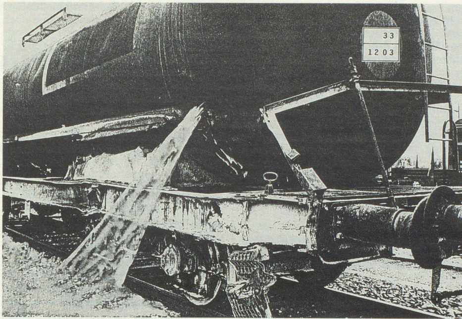
Abb. 3. Die leckgeschlagene Benzinzisterne.
