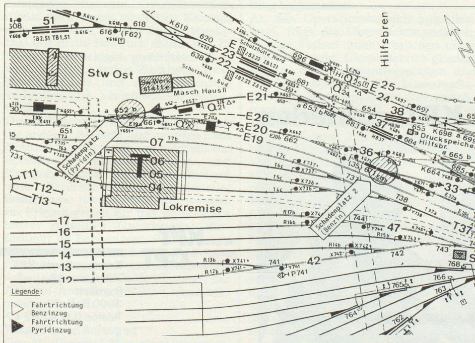
Abb. 4. Situation nach Stillstand der Benzinkomposition.
