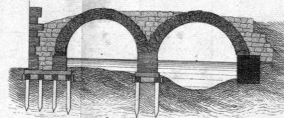
Durchschnitt des Kornhaus-Kanal-Gewölbes nach der Linie FG.
