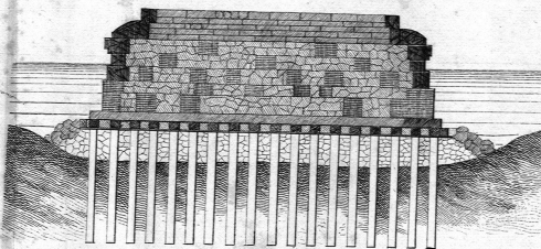
Durchschnitt des Pfeilers III nach der Linie HI.
