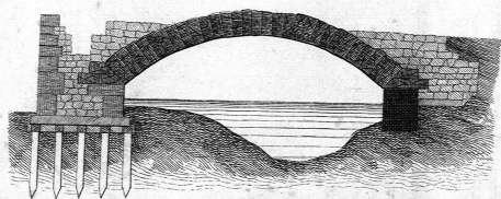
Durchschnitt des Kornhaus-Kanal-Gewölbes nach der Linie DE.
