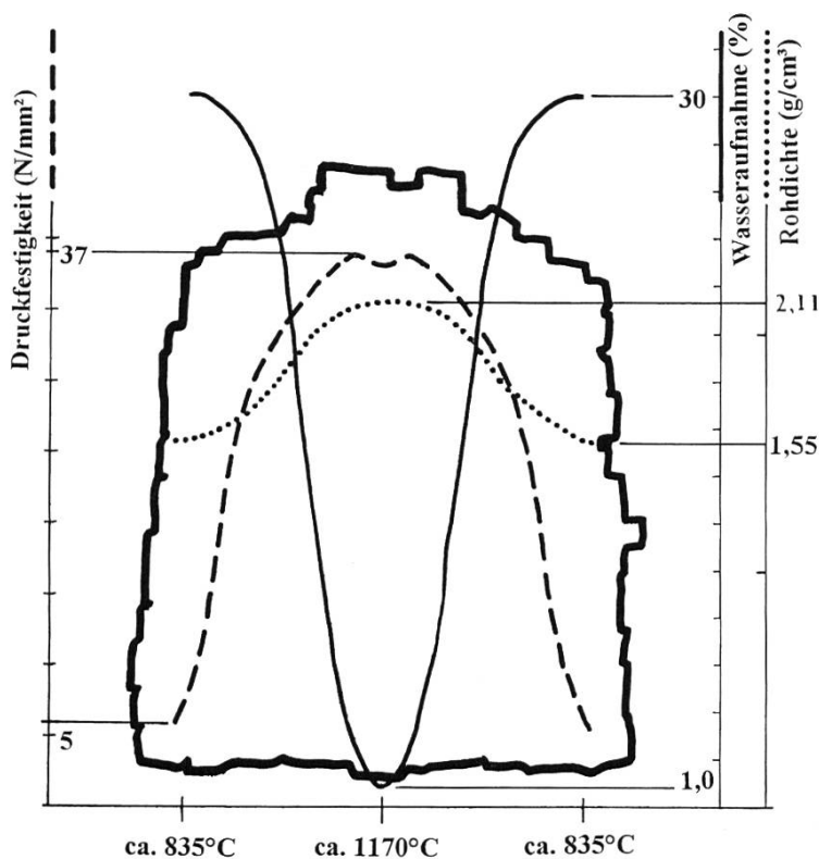
Abb. 7 Nach DIN 105 entspricht diese sortierte Ware einem Vollziegel der Druckfestigkeitsklasse 20–28 N/mm 2 und der Rohdichteklasse 1,8 g/cm 3 .
