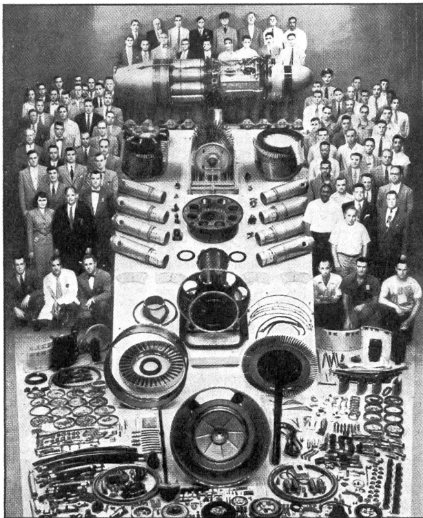
In einer amerikanischen Flugzeugfabrik wird die Herstellung des 10 000. Düsenmotors für Kriegsflugzeuge gefeiert. Das Bild zeigt sämtliche Einzelteile und die gesamte Equipe, die es für die Herstellung eines einzigen solchen Motors braucht.
