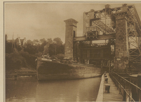
Ein Frachtschiff verläßt den abgesenkten Teil der Schleuse von Hennrichsburg.
