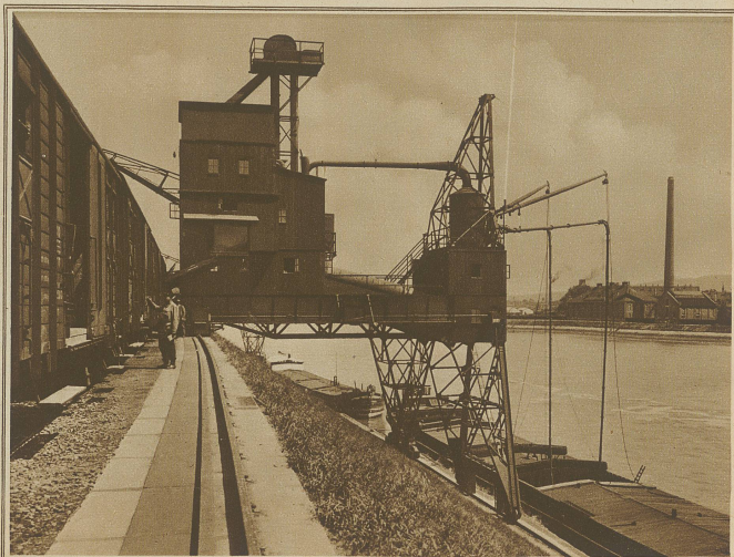
Pneumatischer Getreideheber in Aktion im Hafen von St. Johann, Basel
