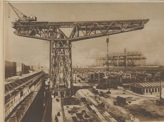
Die größten Drehkrane der Welt befinden sich auf einer Schiffswerft in Hamburg. Der im Bilde ersichtliche Turndrehkran erreicht in hochgehobenem Zustand eine Höhe von über 80 m und ist imstande, 250 Tonnen zu heben
