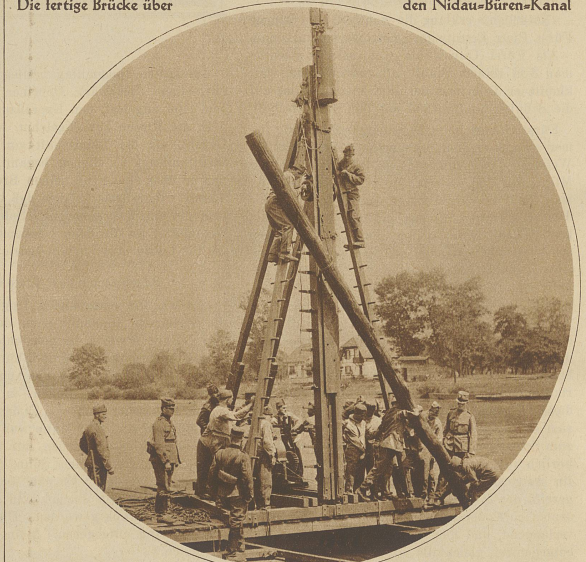
Das Einrammen
