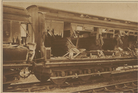
Ein eigenartiges Eisenbahnprojekt ereignet sich in Parkgate bei Rotherham (England). Im Ausgange, als der L. M. S. Express mit 80 km Geschwindigkeit einen Claretzug kreuzte, sprang der letzte freie Kofferwagen aus den Schienen und riss an zwei Wagen des vorbeifahrenden Expresses die Seitenwände heraus, wobei 9 an den Fenstern sitzende Personen getötet wurden
