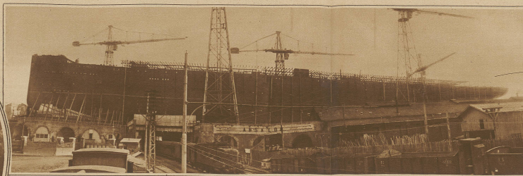
Das größte Motorschiff der Welt. Auf der Ansaldo-Werft in Sestri Ponente bei Genua geht das Motorschiff „Augustus“ seiner Verfertigung entgegen. Es wird mit seinen 3300 Tonnen das größte Motorschiff der Welt (das bisher größte ist das englische „Antares“ mit 2500 Tonnen). Die Länge mißt 215 m bei einer Breite von 25,20 m und Höhe von 15,70 Meter. Das Schiff liegt im Bau quer über der Eisenbahnlinie Genua-Marseille und die Kreuzfahrtschiffe, die diese Straße passieren, müssen nicht, daß sie unter einem Oceanriesen hinwegfahren
