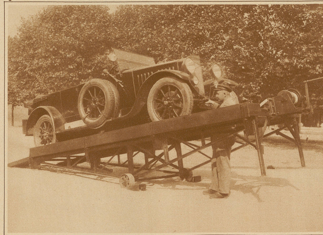
Das Autodock, eine wichtige Erfindung für Automobilisten. Seine Konstruktion erlaubt auch die bequeme Ausführung solcher Reparaturen, die früher nur auf dem Rücken liegend vorgenommen werden konnten
