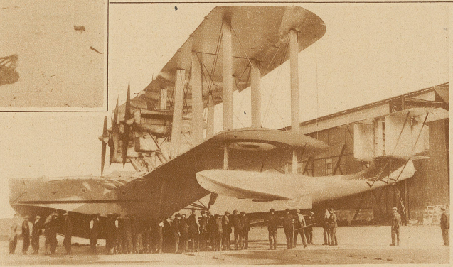
Das größte Wasserflugzeug der Welt ist im Auftrage des englischen Luftverkehrsministeriums für eine Fluglinie London-Indien gebaut worden. Die Motoren entwickeln 2100 P. S.
