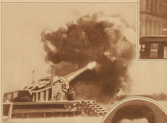
Abschuß eines neu gebauten 16 Zoll Langrohr-Geschützes auf dem Prüffeld von Aberdeen bei Washington. Es ist dies das größte Geschütz, das bis heute gebaut wurde
