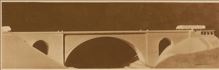
Das Modell der neuen Lorrainebrücke, deren Bau beschlossen wurde und nächstens begonnen werden soll. Die Bauzeit ist auf 2 1/2 Jahre berechnet
