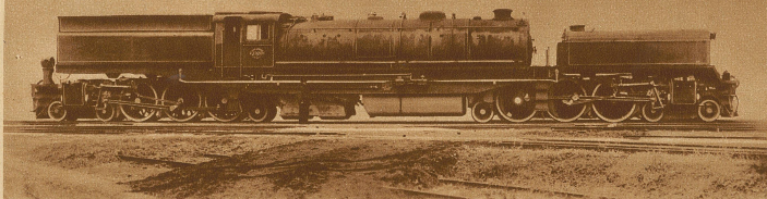
Die schwerste in Europa gebaute 12achsige Lokomotive, die 26,5 m lang ist und 186 Tonnen wiegt. Sie ist für die südafrikanischen Eisenbahnen bestimmt. Das Größenverhältnis veranschaulicht der nahe beim Führerstand stehende Heizer.
