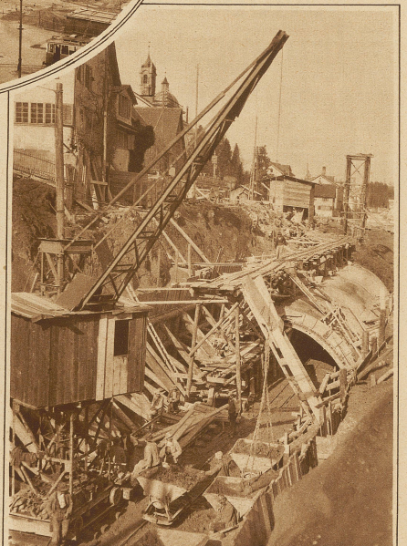
Die Untertunnelung der neuen Bahnlinie längs der Seestraße im Engen-Quartier, zwischen dem neuen Bahnhof und Wollishofen
