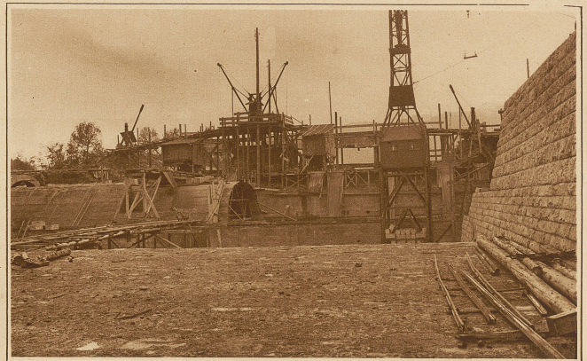
Baukonstruktionen für den quer durch die Sihl führenden Tunnel der neuen Linie
