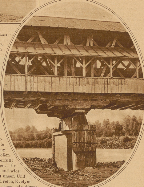
Konstruktionsdetail eines Pfeilers der Brücke bei Ragaz-Maienfeld
