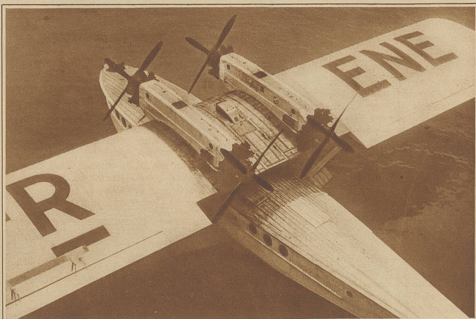
Das neue 4-motorige Großflugboot Dornier-Superwal, das letzte Woche in zwei Stunden von Friedrichshafen über die Alpen nach Genua flog. Das Flugzeug vermag 20 Personen aufzunehmen und erreicht 220 km Höchstgeschwindigkeit in der Stunde
