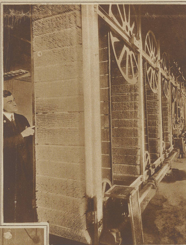
Eine Maschine, die eine Million Streichhölzer auf einmal runde- fertig macht. Wie die Haare einer Bürste, auf einem Bande aufgestellt, tauchen die Hölzchen mit einem Ende in die drei ver- schiedenen Lösungen, die erhärtet das Zündköpfchen bilden
