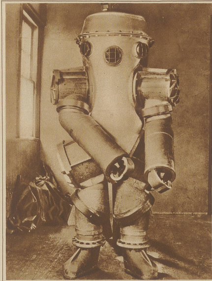
Der eiserne Mensch. Modernster, ganz aus Metall gebauter Taucheranzug, der es ermöglichen soll, bis 100 Meter unter den Wasserspiegel zu tauchen. Man hofft damit wertvolle Funde auf dem Meeresboden machen zu können
