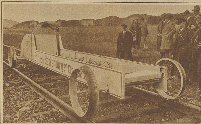
Ein neuer Raketenwagen-Versuch wurde auf der Harzbahnstrecke Blankenburg-Halberstadt unternommen. Das neue Modell hat vorn die Form eines Tropfenautos und ist bedeutend länger gebaut. Es wurden Geschwindigkeiten bis zu 240 km erzielt, aber auch diesmal flog der Wagen aus den Schienen und wurde zertrümmert
