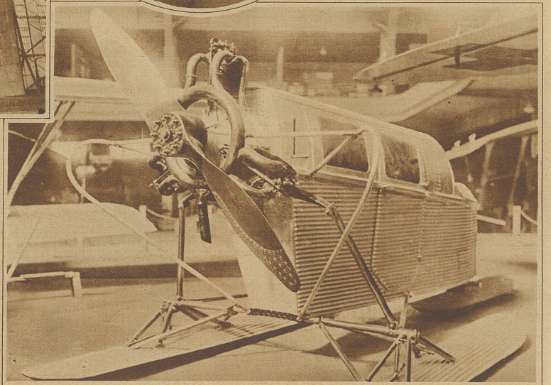
Russischer Motorschlitten mit Propellerantrieb
