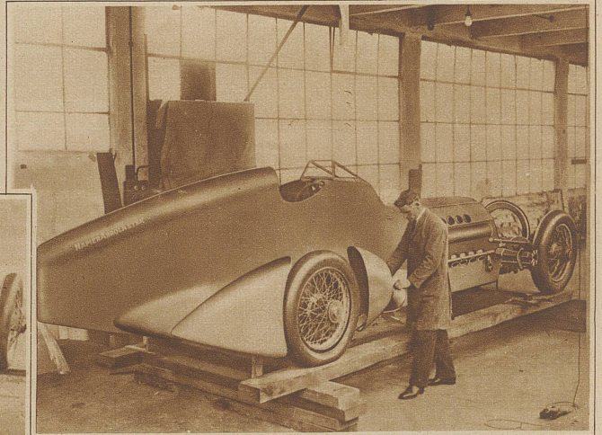
Campbells Rennwagen kurz vor der Fertigstellung in der Werkstatt
