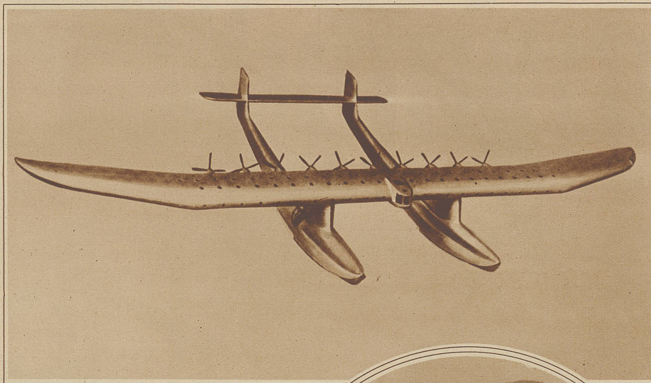
Das Riesenflugzeug der Zukunft. Dr. Edmund Rumpel plant den Bau eines neuen Riesenflugzeuges, das mit 10 Motoren ausgestattet werden soll und 170 Personen faßt. Der Apparat zeichnet sich durch eine ganz neue eigenartige Konstruktion aus. Die zehn 1000 PS-Motoren sind direkt an den Flügeln angebracht, ebenso befinden sich die Passagier- und Führer-Räume in den Flügeln. Für die große Sicherheit des Flugbootes bürgt die Tatsache, daß von den 10 Motoren ohne weiteres 4-5 versagen können, ohne daß die Flugfähigkeit des Apparates darunter leidet. Das Flugboot, dessen Modell unser Bild zeigt, ist für 135 Passagiere und 35 Mann Besatzung vorgesehen.
