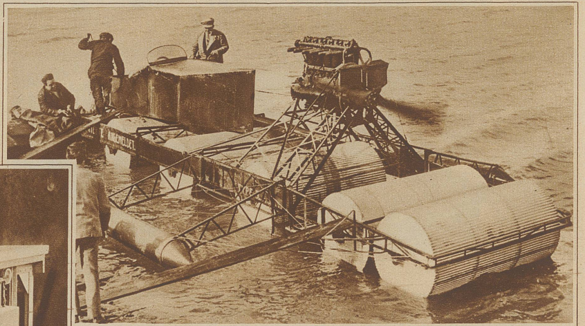
Ein neuartiges Wasserfahrzeug machte dieser Tage in Wien seine erste erfolgreiche Probefahrt. An Stelle des Schiffsrumpfes besitzt das Fahrzeug rotierende Hohlzylinder; der Antrieb erfolgt durch einen Propeller mit einem 200 PS Flugzeugmotor
