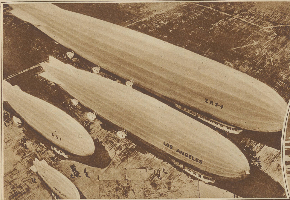
Links: Amerika baut neue Luftriesen. Graphische Darstellung der kleinsten und der größten lenkbaren Luftschiffe der amerikanischen Marine. Welch gewaltige Ausmaße der im Bau begriffene «Z. R. S - 4» hat, zeigt ein Vergleich mit der danebenstehenden «Los Angeles», die in ihrer Größe ungefähr dem in Friedrichshafen gebauten «Graf Zeppelin» entspricht. Gleichzeitig mit dem «Z. R. S - 4» wird ein gleich großes Schwesterschiff «Z. R. S - 5» gebaut
