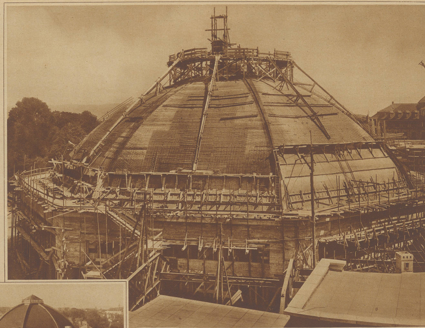
Nebenstehendes Bild: Die Eisenbetonkuppel der Markthalle Basel
