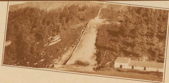
Die neue Maloja-Skisprungschanze im Bau. Die riesige Anlage, deren Ausmaße diejenigen aller bestehenden Schanzen weit übertreffen, ist in technischen Fachkreisen stark umstritten, vor allem dort, wo man findet, die Rekordsucht sollte nicht weiter gefördert werden. Erbauer der Schanze ist der bekannte Skispringer Badrutt, der die Arbeit ohne irgendwelche Pläne und Berechnungen ausführt (Phot. Bucher)
