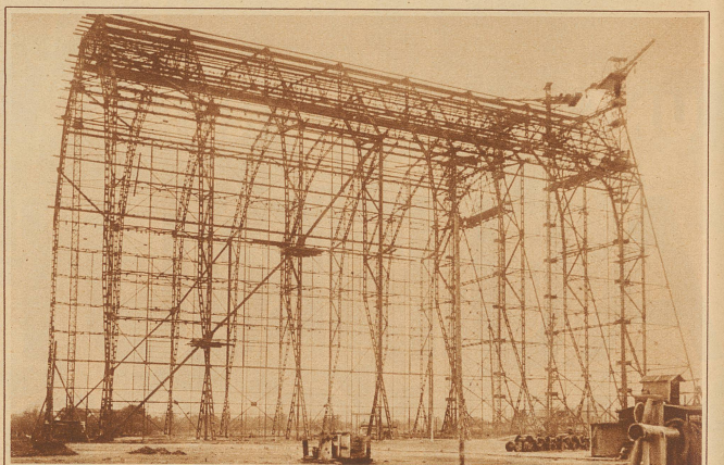
Die größte Luftschiffhalle der Welt mit 900 000 Kubikmeter umbautem Raum ist gegenwärtig in Friedrichshafen im Bau begriffen. Sie soll schon im März nächsten Jahres fertig sein und zur Aufnahme des neuen riesigen Zeppelinluftschiffes dienen
