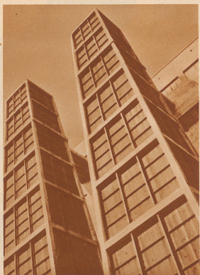
Die Dunstabzugsschächte der Gaskokerei in Schlieren. Sie sind 32 m hoch und bilden jetzt mit dem 72 m hohen Hochkamin und dem Kohlenturm die Dominante des umgebauten Werkes
