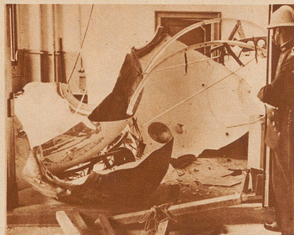
Cosyns Stratosphärengondel explodiert. In der Universität Brüssel ist die Gondel, mit der Cosyns in den nächsten Tagen einen neuen Stratosphärenflug unternehmen wollte, im Verlauf der Probe auf ihre Druckwiderstandskraft explodiert. Ein Arbeiter wurde getötet. Cosyns blieb unverseht
