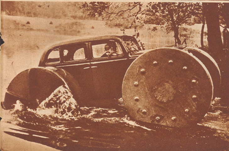
Das Wasserauto geht an Land. Der Kölner Erfinder Walter Bodenstein hat in diesen Tagen die ersten Versuche mit einem von ihm konstruierten Wasserauto gemacht. An Stelle der normalen Räder sind am Wagen vier Pontonräder montiert, die Schwimmkörper und Wasserantrieb zugleich darstellen. Das vordere Räderpaar dient als Steuer, das hintere — es sind Schaufelräder — bewirkt die Fortbewegung. Wie groß die praktische Verwendbarkeit dieser neuen Erfindung ist, muß die Zukunft lehren.
