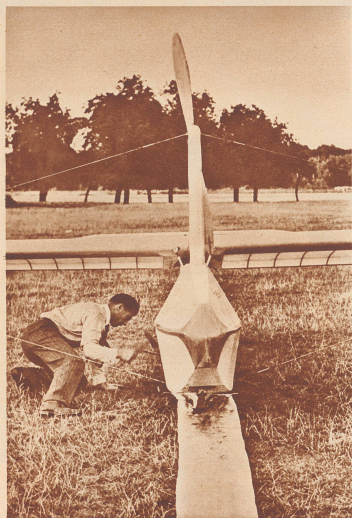
Räder besitzt das Muskelkraftzeug nicht, es startet mit einer Kufe auf einer gerigten Gleitbahn und landet wie ein Segelflugzeug. Das Bild zeigt einen der Konstrukteure, Haessler, beim Einschlagen des Hakens, der die Maschine bis zum Start festhält.
