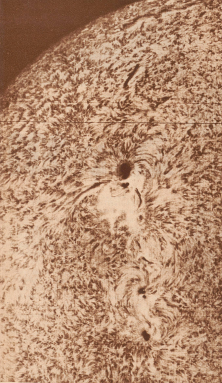
Teil der Sonnenoberfläche, aufgenommen im Lichte des Sonnenrotes. Die Wirbelbildung in der Umgebung der Sonnenflecken ist besonders deutlich. Aufnahme von der Mt. Wilson-Sternwarte in Kalifornien.
