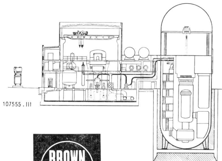
Schnitt durch das Atomkraftwerk
