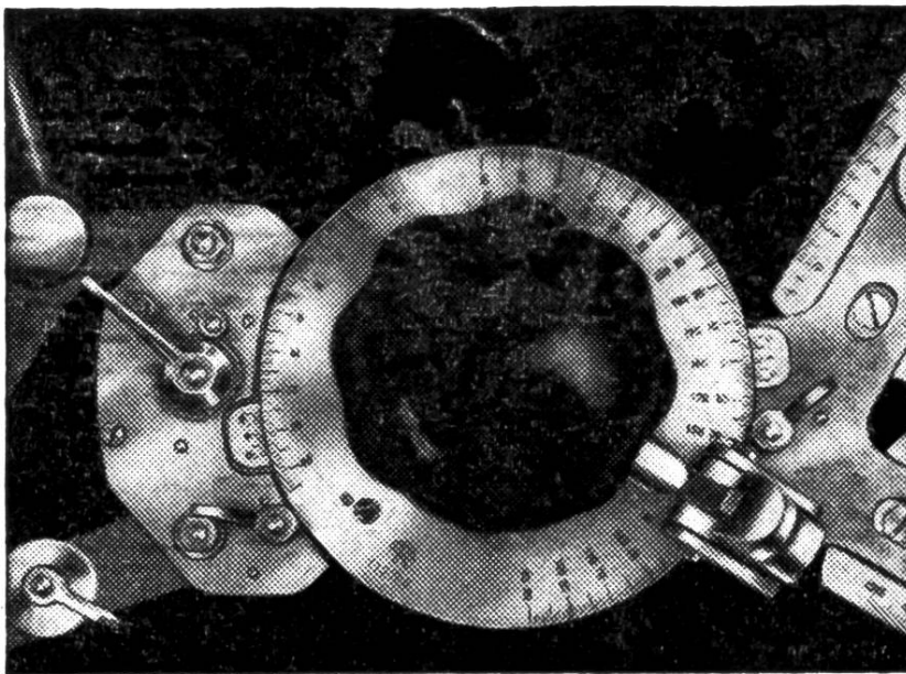
Kuhlmann-Zeichenkopf mit Basisverstellung
