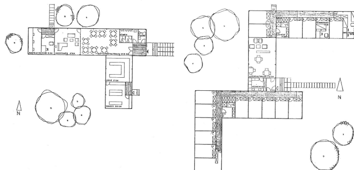
Grundriss eines Gemeinschaftspavillons und eines Bettenpavillons.
