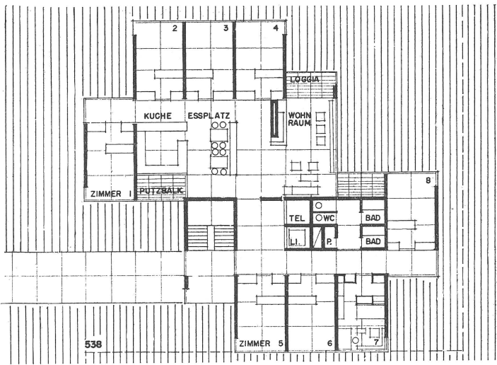
Wohngruppe für Ledige mit 8 Einzimmer, zentralem Wohnraum und Küche. Projekt Kapp.
