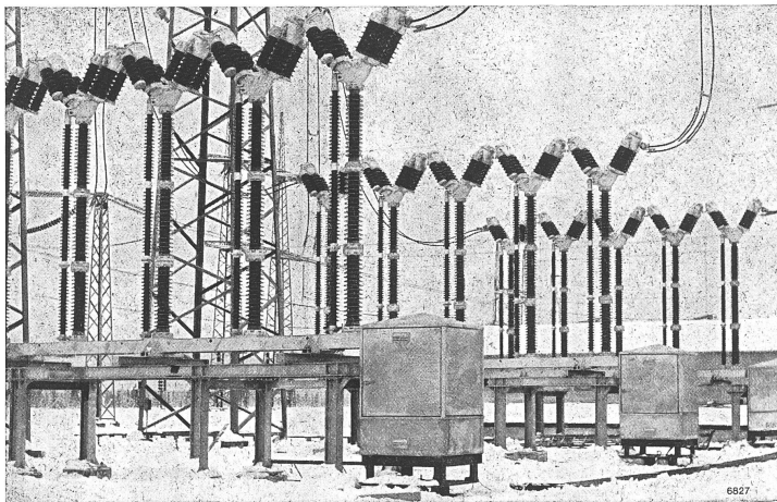
Oelarmar Leistungsschalter mit Mehrfachunterbrechung für 420 000 V, in Kilforsen, Schweden
