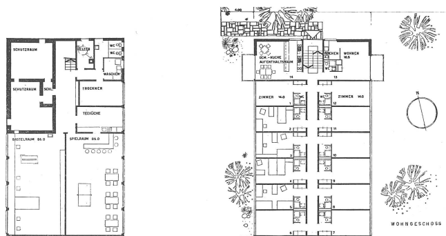
Grundriss Wohngeschoss und Kellergeschoss des Projektes Altstetten. Entwurf Architekt F. Hodler
