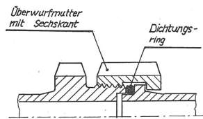
Figur 2 Das Gewinde ist links direkt ins Rohrmaterial geschnitten. Mit einer Überwurfmutter wird das rechte Rohrende an das linke gepresst. Ein Kautschukring dient als Dichtung.
