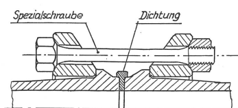
Figur 4 Gleiches Prinzip wie in Figur 3. Die Flanschen hat man sich hier als lose Ringe vorzustellen. Die Dichtung übernimmt ein Ring aus weichem Metall.
