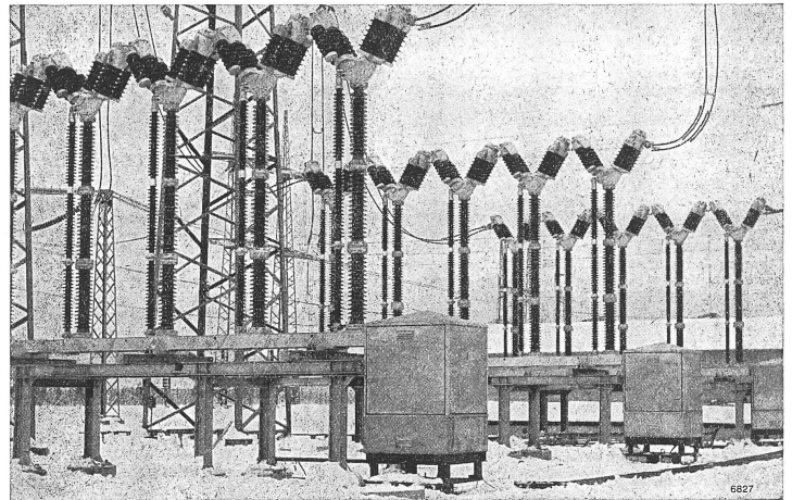
Oelarmierter Leistungsschalter mit Mehrfachunterbrechung für 420 000 V, in Kilförsen, Schweden
