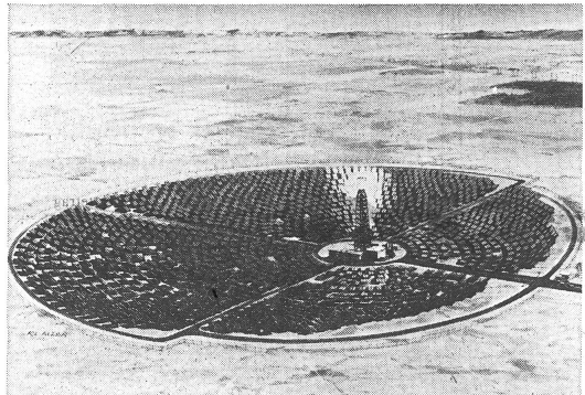
Die amerikanische Sonnenzentrale im kalifornischen Brawley soll einmal mit 1800 Spiegeln, die elektronisch gesteuert, ihren Brennpunkt ständig auf den Wasserbehälter in hundert Meter Höhe im Zentrum des Spiegelparks richten, arbeiten. Mit einer Jahresleistung von 10 Megawatt kann dieses Werk eine Kleinstadt von 10 000 Einwohnern mit Energie versorgen.
